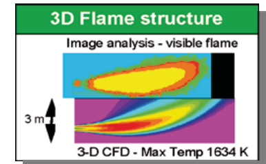
Modélisation des feux et des explosions.
