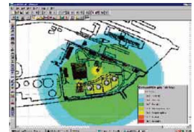
Évaluation des contours de risque (BLEVE, JetFire...)
