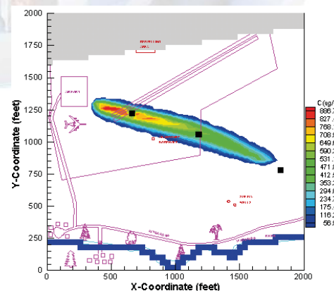
Simulation de l'étendue d'une pollution de sol.
